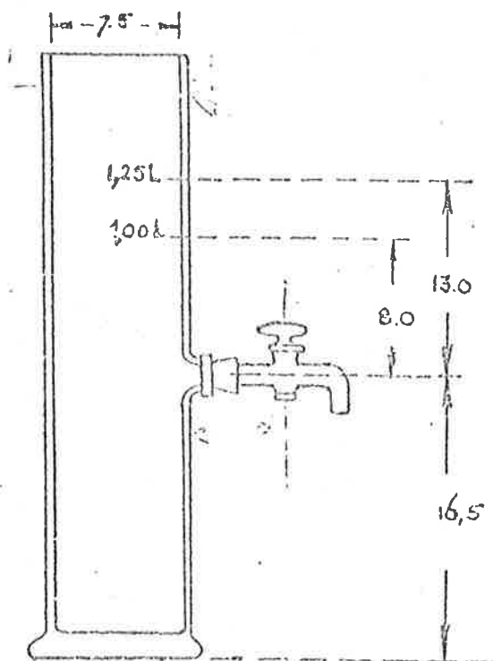
FIG. 2 (1/4 nat. grootte) Sedimentatie-cylinder - Kraanboring 7 mM.
